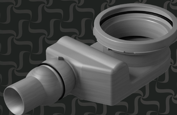
S baza sa 28mm vodenog čepa i podesivim izlazom
